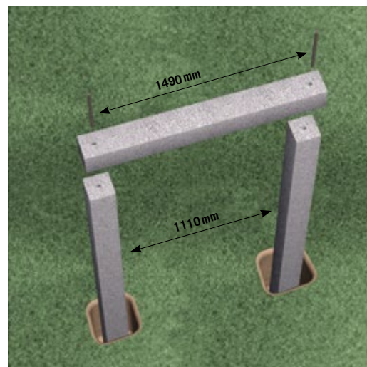
De stående balkarna förankras ordentligt i marken.
