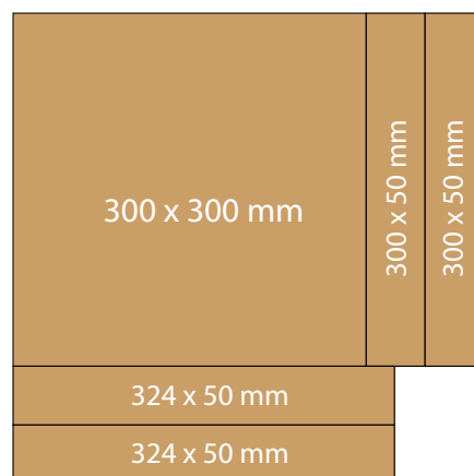
Såga delarnas storlek enligt denna ritning.
